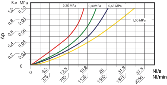
Diagrammet viser ulike inngangstrykk inntil trykkfall maks. 1 bar
