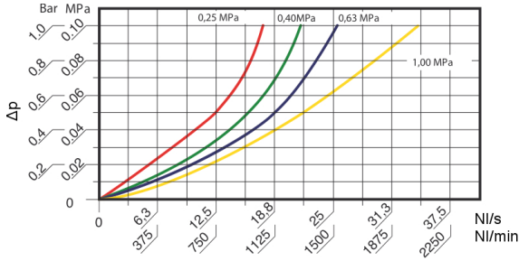
Diagrammet visar olika ingångstryck upp till tryckfall max. 1bar
