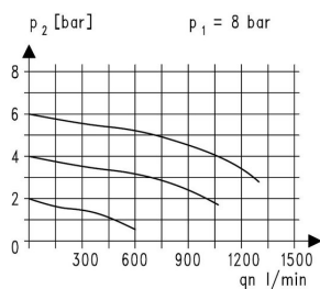
Flödesdiagramm
