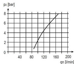
Olieforstøverens aktiveringsgrænse
