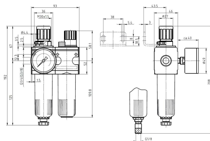
halvautomatisk tappeventil
