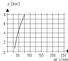
Oljeapparatets aktiveringsgrense
