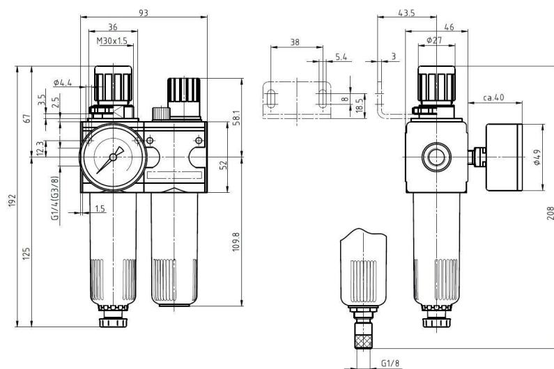
halfautomatische aftapkraan
