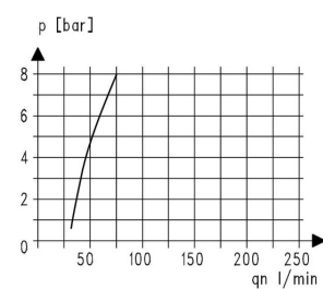
Olievernevelaar-inschakeldrempel
