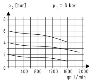
Doorstroombiagramma
