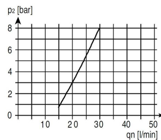
Öljysumuttimen toimintaraja
