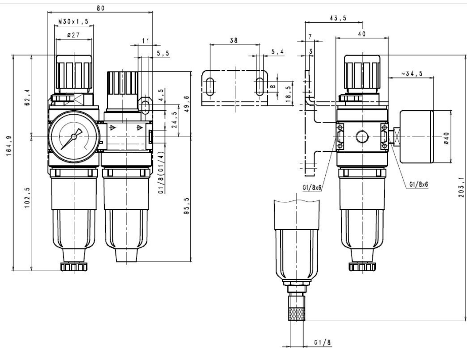
puoliautomaattinen tyhjennysventtiili
