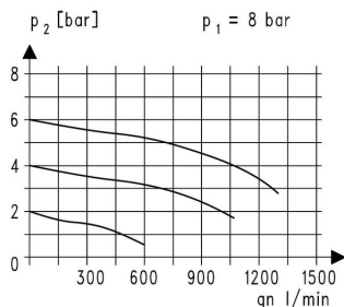
Strömungsdiagramm
