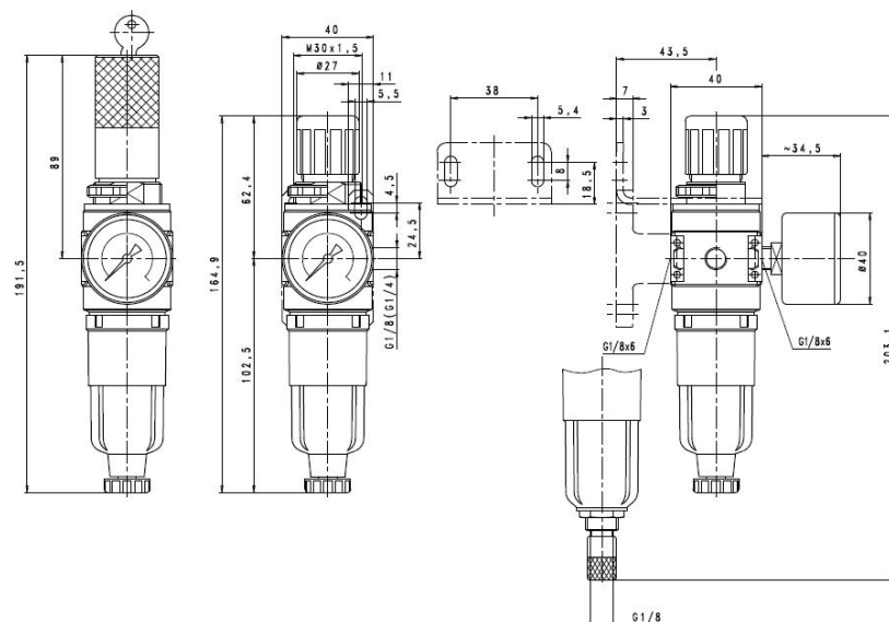
halvautomatisk aftapningsventil
