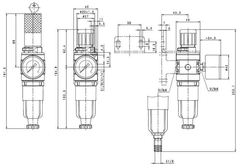
purgeur semi-automatique
