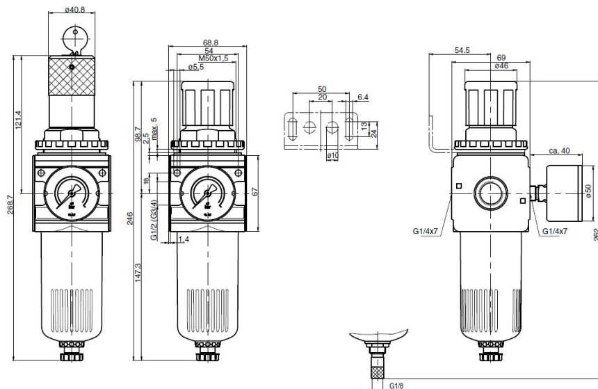
puoliautomaattinen tyhjennysventtiili
