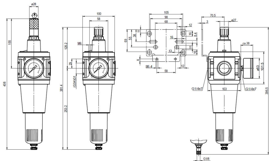
valvola di scarico semiautomatica valvola di scarico automatica
