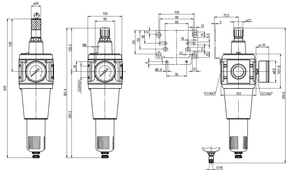
puoliautomaattinen tyhjennysventtiili tyhjennysventtiili automaattinen
