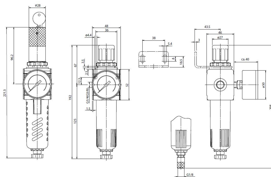
valvola di scarico semiautomatica
