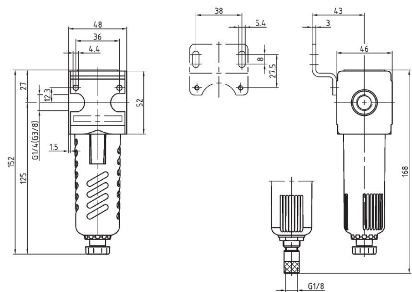
purgeur automatique
