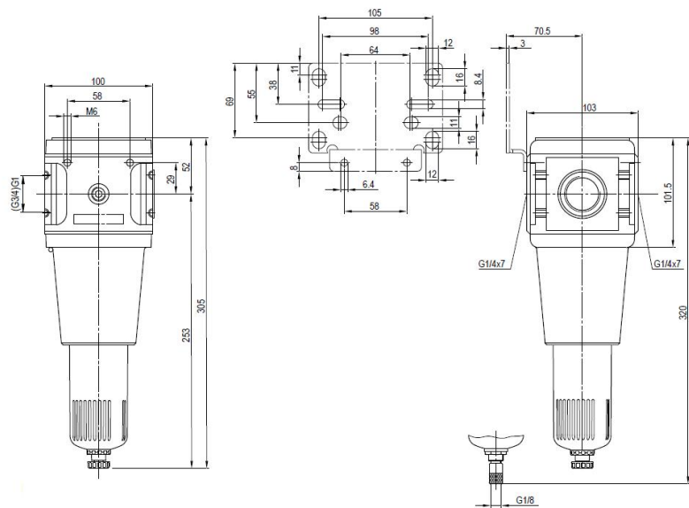
automatisk aftapningsventil
