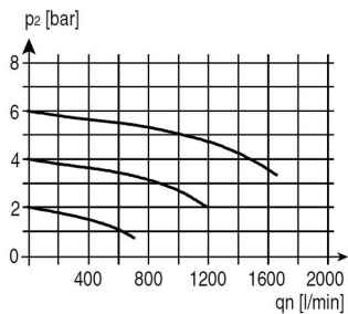
Diagrama de caudal
