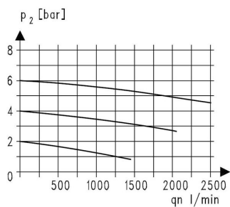
Virtauskaavio
