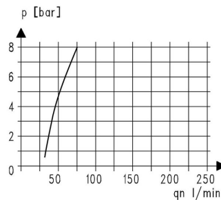
Öljysumuttimen toimintaraja
