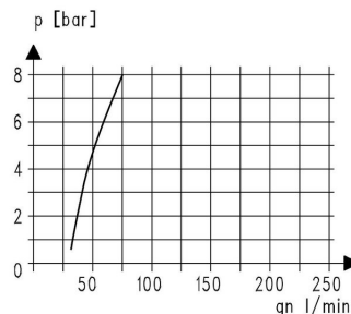
Öljysumuttimen toimintaraja
