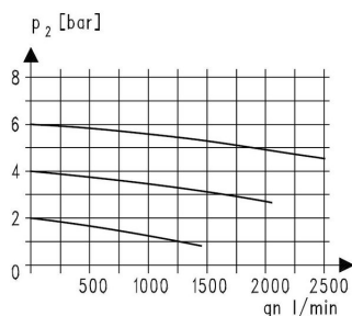
Virtauskaavio
