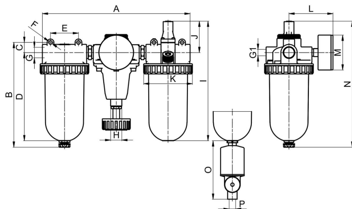
automaattinen tyhjennysventtiili
