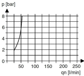
Soglia di intervento dell'oliatore
