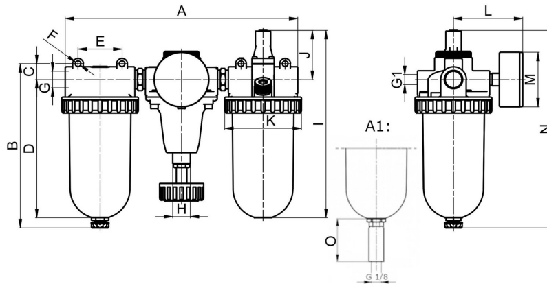
A1: valvola di scarico automatica
