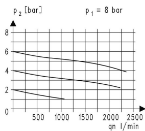
Wykres przepływu
