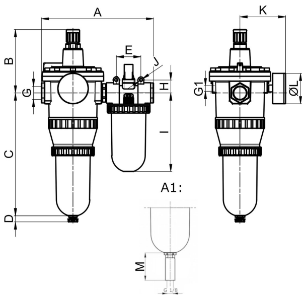
A1: válvula de purga automática
