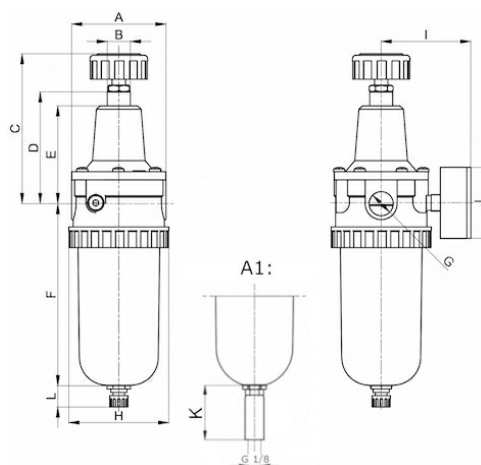
A1: αυτόματη βαλβίδα αποστράγγισης
