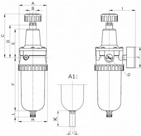
A1: purgeur automatique
