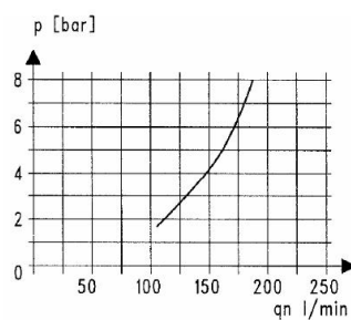
Öljysummittimen toimintaraja
