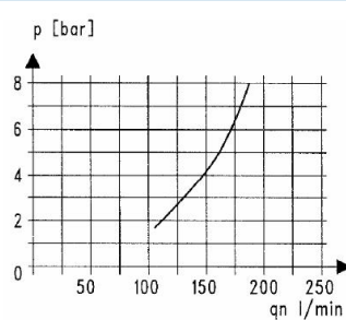
Öljysumuttimen toimintaraja
