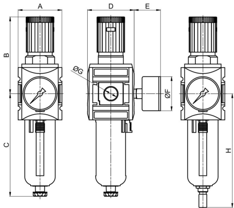
purgeur semi-automatique
