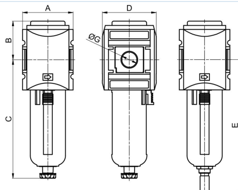
halvautomatiskt avtappningsventil
