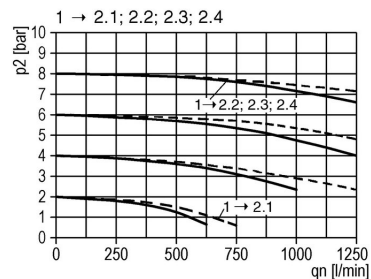
2. Strømningsdiagramm
