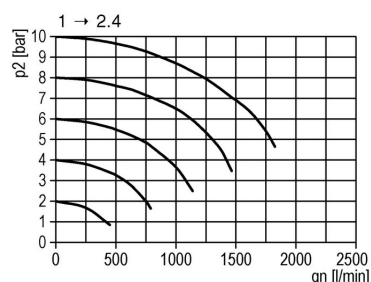
2. Strømningsdiagramm
