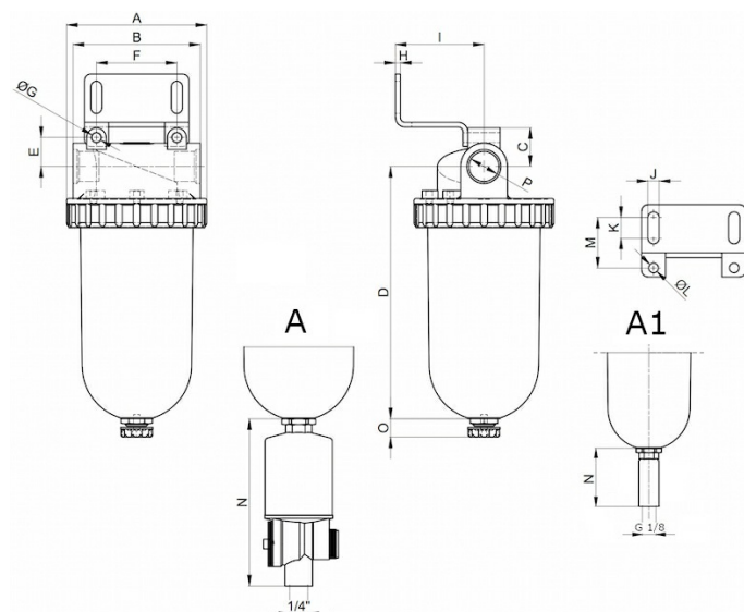
A, A1: automatisk aftørningsventil
