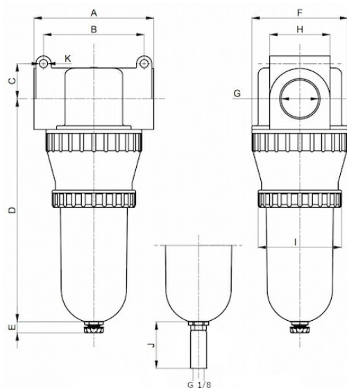
automatski ispusni ventil
