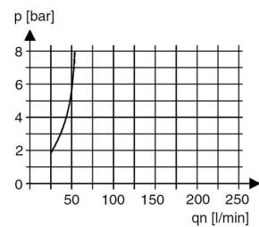
Öljysumuttimen toimintaraja
