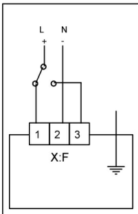
Commande 3 points
