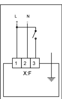
Commande 2 points
