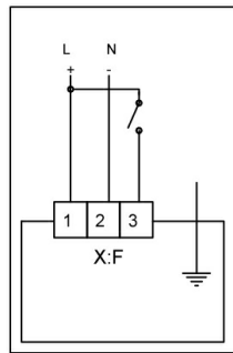
2-punktsstyrning
