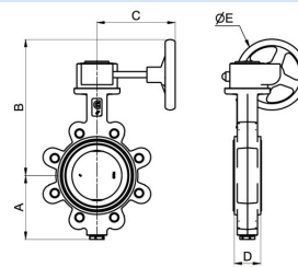
Έκδοση με φλάντζα σύνδεσης
