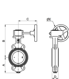
Međuprostavna izvedba priрубnice
