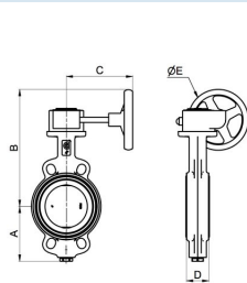
Tussenflensuitvoering
