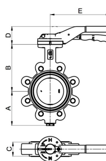
Flänsutförande
