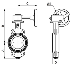
Mellemflangeudførelse
