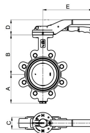
Prirubnička izvedba
