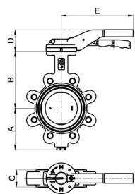
Versión con brida
