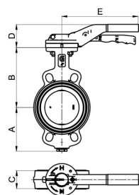
Versión con brida intermedia
