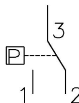
Διακόπτης κενού
