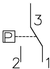
Διακόπτης πίεσης
