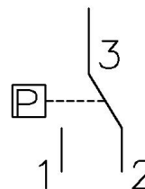
Vakuumbryter
