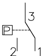
Trykkbryter
