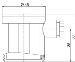
Consolă de fixare Tip 6403
