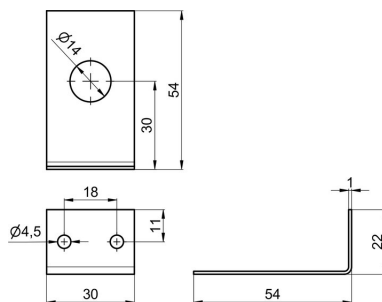
Consolă de fixare Tip 6403
