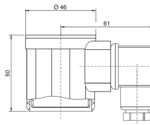
Capac de protecție cu priză de aparat IP65 Tip 6379
