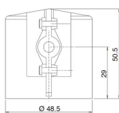
Capac de protecție IP44 Tip PC-PVS01-01
