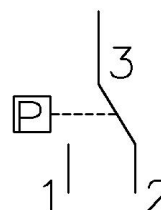
Comutator de vid
