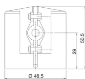
Capac de protecție IP44 Tip PC-PVS01-01
