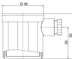
Skyddskåpa med PG-förskruvning Typ 6371 (IP54) / 6372 (IP65)
