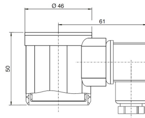
Skyddskåpa med apparatuttag IP65 Typ 6379
