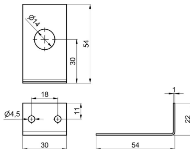
Monteringsvinkel Typ 6403
