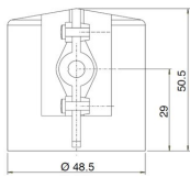
Skyddshätta IP44 Typ PC-PVS01-01
