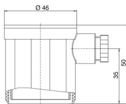
Suojakupu PG-kaapeliläpiviennillä Tyyppi 6371 (IP54) / 6372 (IP65)
