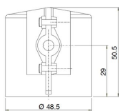
Suojakuppi IP44 Tyyppi PC-PVS01-01
