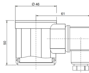
Suojakupu laitepistorasialla IP65 Tyyppi 6379
